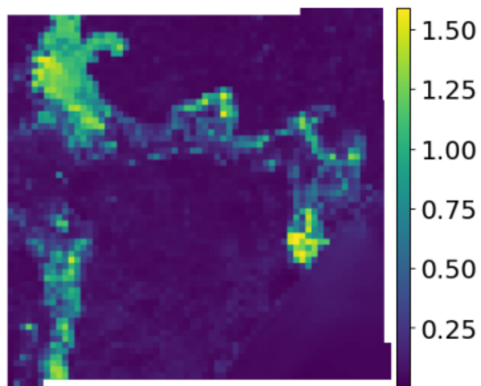
Cosine baseline
