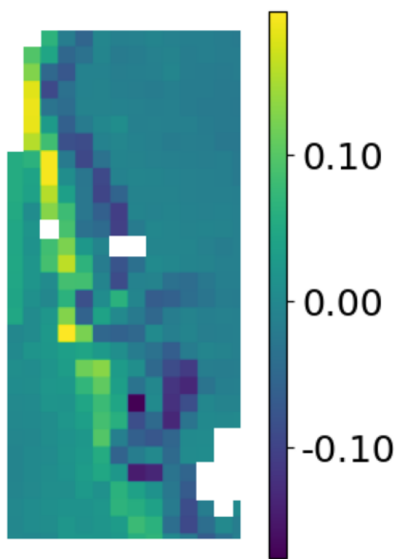
NDVI
