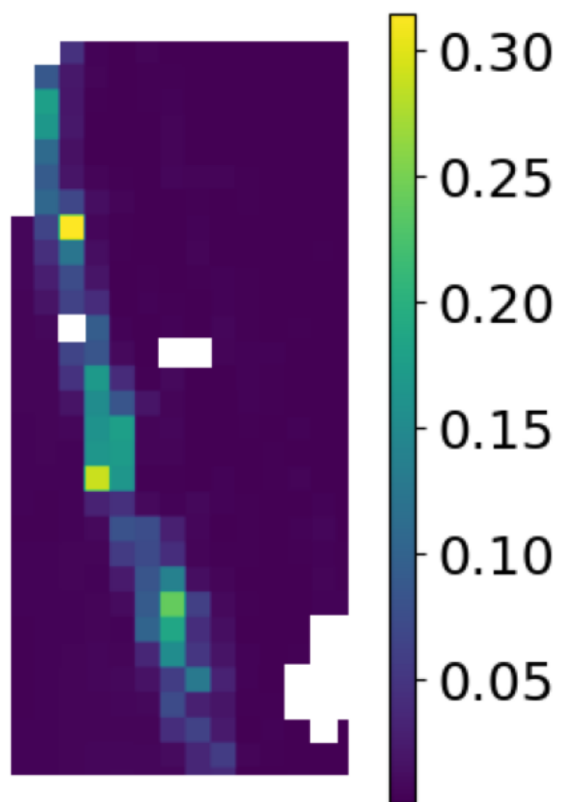
Cosine baseline
