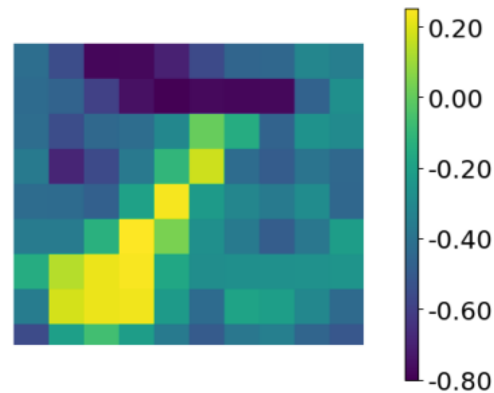
NDVI
