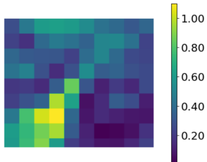
Cosine baseline
