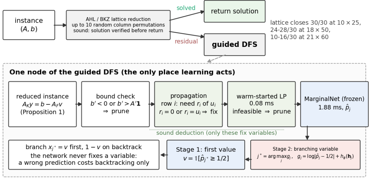
그림 1. 배포 시스템. lattice 단계가 먼저 돌아 성공하면 검증된 해를 반환하고, guided depth-first search는 그 잔여를 본다. 탐색 node 안에서 변수를 확정하거나 가지를 치는 것은 건전 추론(bound 검사, propagation, relaxation의 infeasibility 판정)뿐이고, 학습 컴포넌트는 분기할 변수와 먼저 시도할 값만 고른다. 동결된 marginal network가 \hat{p}_j 를 내고 Stage 1은 거기서 값을, Stage 2는 비용으로 조정된 policy head에서 변수를 취한다. 어느 쪽도 변수를 확정하지 않으므로 잘못된 예측의 대가는 backtracking뿐이다.
