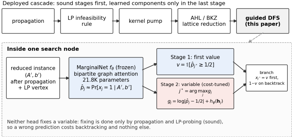
그림 1. 배포 시스템과 두 학습 컴포넌트. cascade는 건전한 단계를 먼저 돌리고 학습 컴포넌트는 마지막 guided depth-first search 안에서만 작동한다. 한 node에서 동결된 marginal network가 \hat{p}_j 를 내고, 먼저 시도할 값은 \hat{p}_j 에서(Stage 1), 분기할 변수는 비용으로 조정된 policy head에서(Stage 2) 나온다. 어느 쪽도 변수를 확정하지 않는다.
