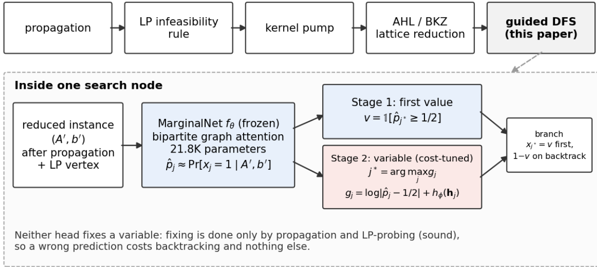
그림 1. 배포 시스템과 두 학습 컴포넌트. cascade는 건전한 단계를 먼저 돌리고 학습 컴포넌트는 마지막 guided depth-first search 안에서만 작동한다. 한 node에서 동결된 marginal network가 p^\wedge 를 내고, 먼저 시도할 값은 p^\wedge 에서(Stage 1), 분기할 변수는 비용으로 조정된 policy head에서(Stage 2) 나온다. 어느 쪽도 변수를 확정하지 않는다.
