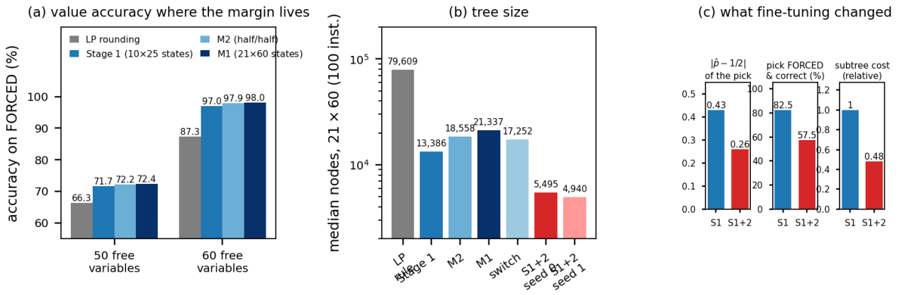
그림 8. 값 정확도와 tree 크기는 독립적으로 움직인다. (a) 자유 변수 50개와 60개인 21×60 in-tree 상태의 FORCED 변수 정확도: relaxation rounding, 10×25 상태로 학습한 Stage 1 network, 같은 architecture를 21×60 상태(M1)나 반반 혼합(M2)으로 학습한 것. (b) 100개 세트의 node 중앙값: 값 정확도가 높은 network가 node를 더 많이 전개하고 비용으로 조정된 policy는 덜 전개한다. (c) held-out 상태 300개에서 fine-tuning된 policy는 덜 확신하는 변수, FORCED이면서 맞는 경우가 더 적은 변수를 고르고 그 subtree 비용은 절반이다.
