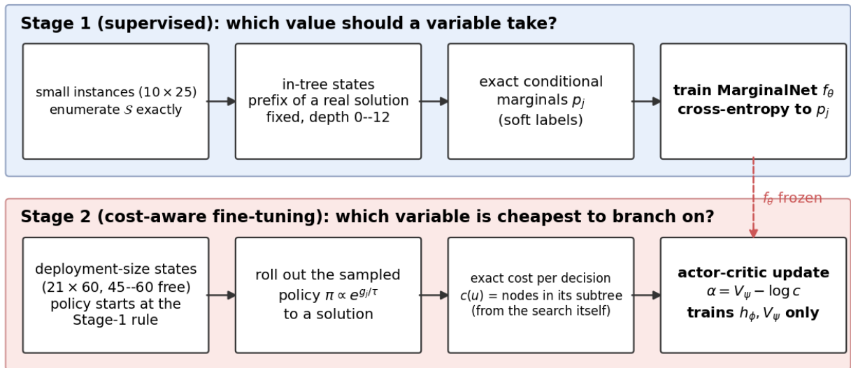
그림 3. 두 학습 단계. Stage 1은 열거 가능한 instance의 정확한 conditional marginal에서 어느 값을 배우고, Stage 2는 탐색이 산출하는 모든 결정의 정확한 subtree 비용에서 어느 변수를 배운다. Stage 1 network는 동결된다.
