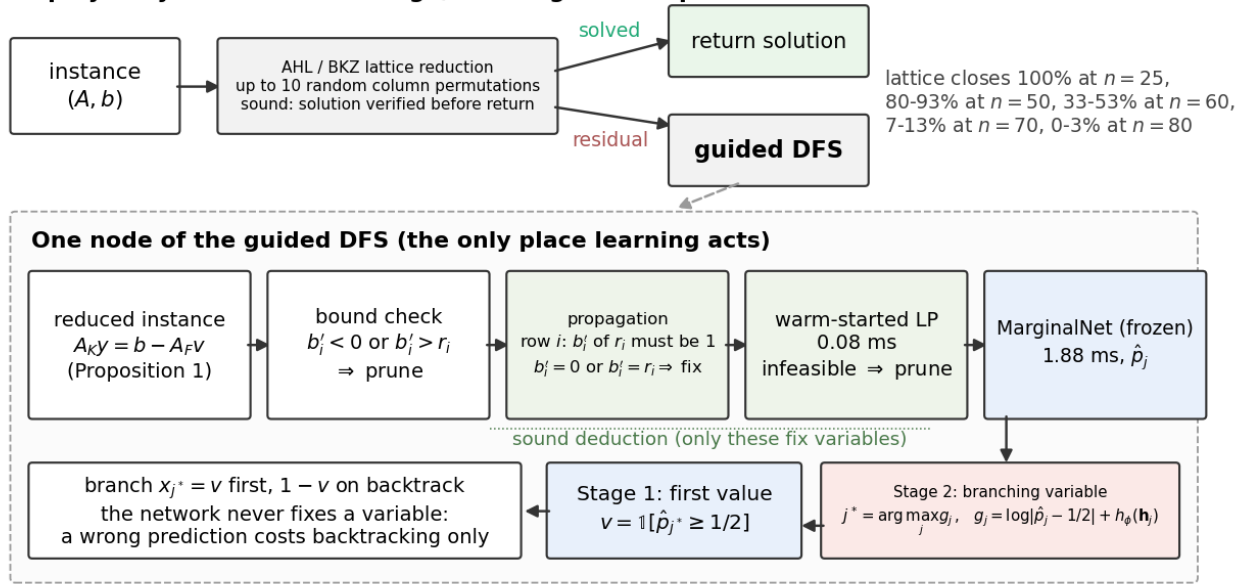
그림 1. 배포 시스템. lattice 단계가 먼저 돌아 성공하면 검증된 해를 반환하고, guided depth-first search는 그 잔여를 받는다. node 안에서 변수를 확정하거나 가치를 치는 것은 건전 추론(bound 검사, propagation, relaxation infeasibility)뿐이고 학습 컴포넌트는 분기 변수와 먼저 시도할 값을 고른다. 동결된 marginal network가 \hat{p}^\Delta 를 내고, Stage 1은 거기서 값을, Stage 2는 비용으로 조정된 policy head에서 변수를 취한다. 잘못된 예측의 대가는 backtracking뿐이다.
