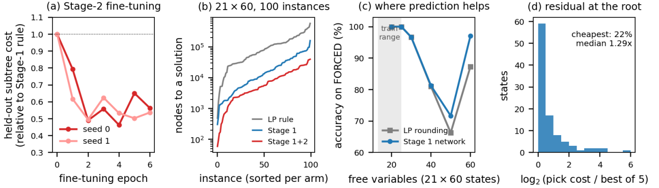
그림 5. (a) Stage 2 fine-tuning: held-out 상태 150개의 총 subtree 비용(Stage 1 규칙 대비), 학습 seed 둘; 선택된 epoch는 4와 2. (b) 21 \times 60 100개 세트에서 해까지의 node 수, arm별 정렬. (c) 21 \times 60 in-tree 상태의 FORCED 변수 정확도(자유 변수 수별): Stage 1의 relaxation rounding 대비 마진은 학습 범위 밖에 있다. (d) root의 잔차: 확신도 규칙 선택의 비용을 후보 5개 중 가장 싼 것 대비로(held-out 상태 100개, 자유 변수 45~50).
