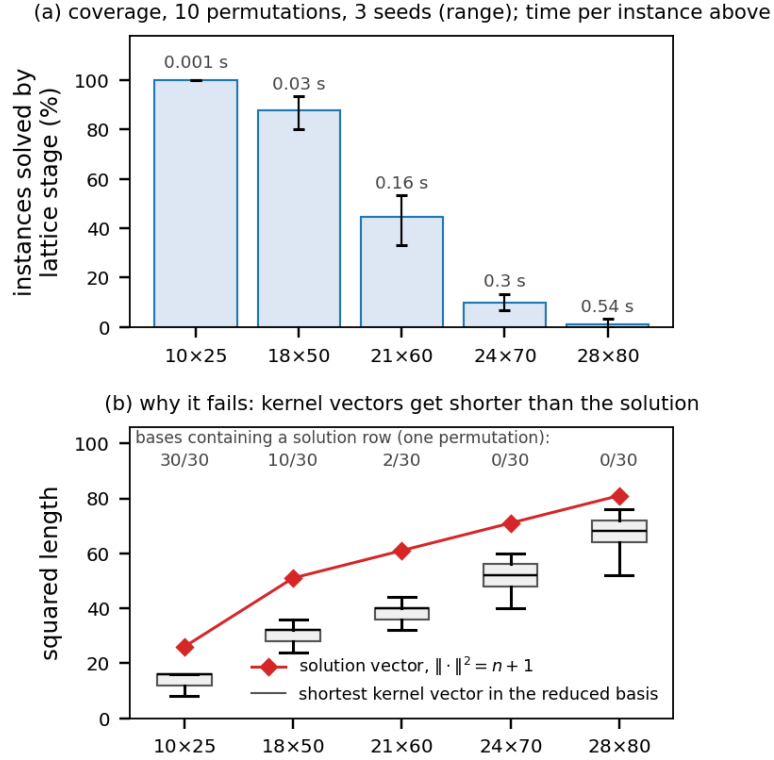
그림 4. lattice 단계. (a) 열 순열 10개, seed 3개로 푸는 instance 비율(막대: 평균, whisker: 범위; 위의 숫자: instance당 시간 중앙값). (b) 축약 기저의 가장 짧은 kernel형 vector의 길이 제곱(instance 30개, 순열 1개의 box)과 해 vector의 길이 제곱 n+1 ; 위의 숫자는 축약 기저에 해 행이 포함된 instance 수.
