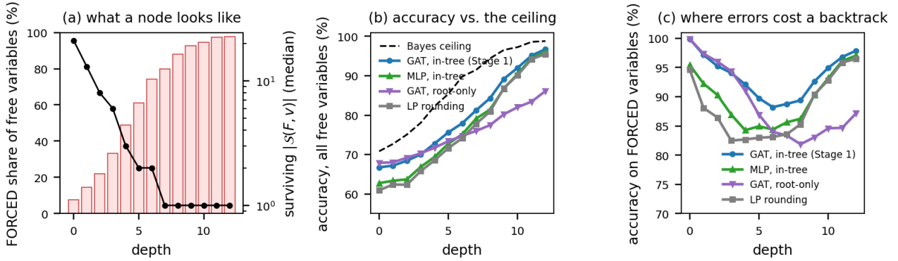
그림 7. 10 \times 25 instance의 held-out in-tree 상태 2,640개에서 정확한 posterior 대비 예측, depth별. (a) 자유 변수 중 FORCED 비중과 살아남은 해 수의 중앙값. (b) 모든 자유 변수에 대한 변수별 정확도와 Bayes 상한 (3). (c) 오류가 backtrack 비용을 낳는 FORCED 변수에서의 정확도. 네 predictor는 라벨·손실·상태를 공유한다: Stage 1 network(in-tree로 학습한 GAT), root 상태만으로 학습한 같은 GAT, in-tree로 학습한 제약 집계 특징의 graph-free MLP, relaxation rounding.
