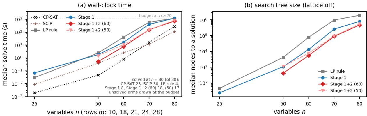
그림 6. 크기에 따른 스케일링(표 3). (a) wall-clock 시간 중앙값; n \geq 70 에서 whisker는 seed 3개의 범위이고 n=80 의 미해결 arm은 예산에 그렸다(해결 수는 안에 표기). (b) 해까지의 node 중앙값, lattice off. 두 단계 모두 n \leq 60 에서 학습했다.
