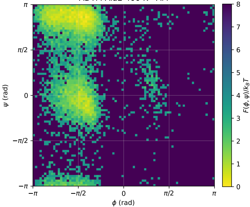
ADTM Ala2 400 K - AM
