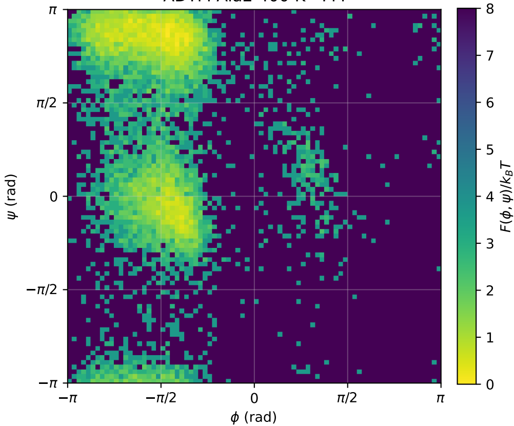
ADTM Ala2 400 K - FM
