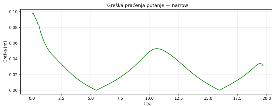
Slika 6.9. Greška praćenja u scenariju uskog prolaza. Dva područja povišene greške odgovaraju dvjema najizraženijim krivinama putanje.
