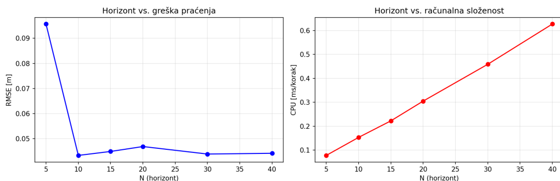
Slika 6.22. Greška praćenja (RMSE) i prosječno CPU vrijeme u ovisnosti o predikcijskom horizontu N . Zadana vrijednost N = 20 označena je kao referentna.
