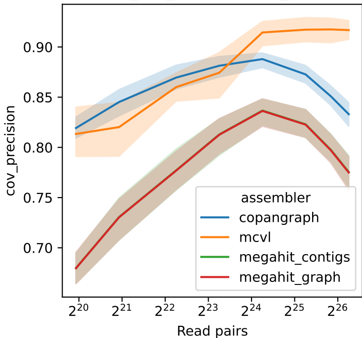
megahit_cov_precision cov_precision
