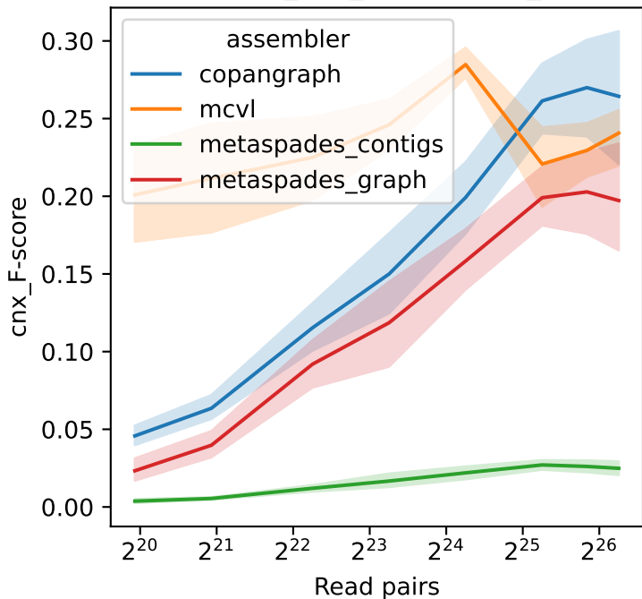
metaspades_cnx_F-score cnx_F-score
