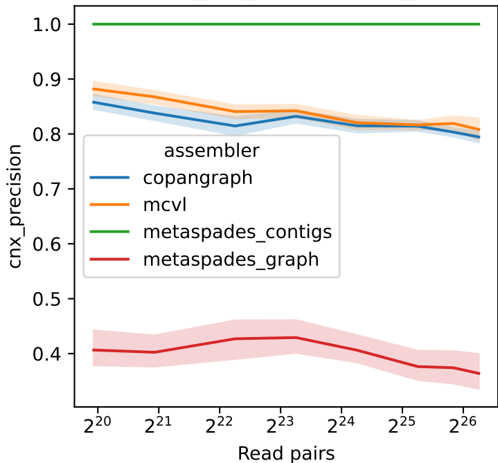
metaspades_cnx_precision cnx_precision
