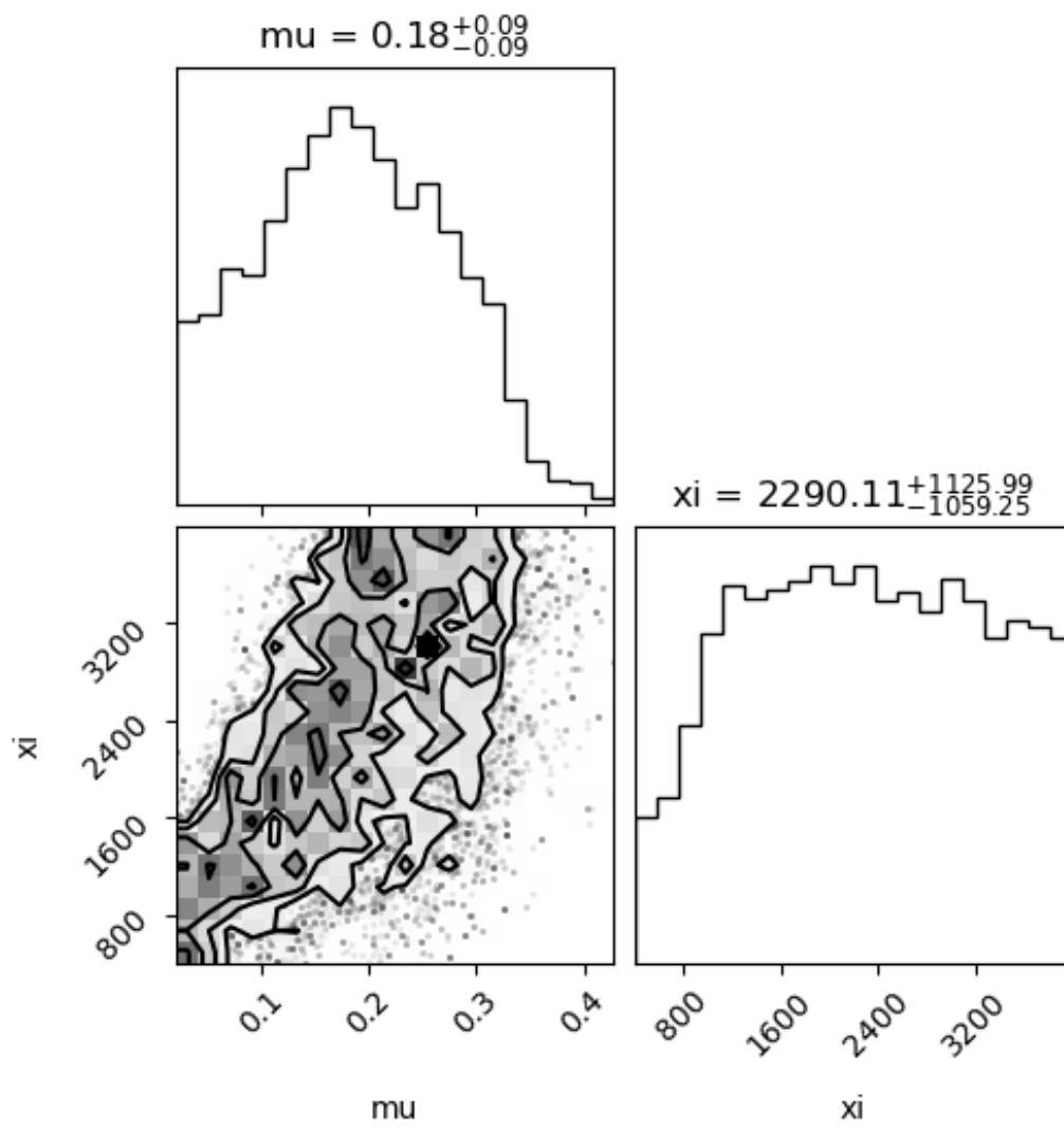
Figure 1 - Pairwise posterior corner plot.
