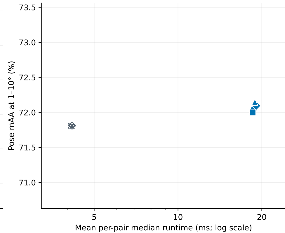
ALIKED-LightGlue · 70 pairs / 7 scenes · 1.5 px
