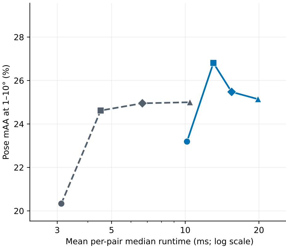
SIFT · 70 pairs / 7 scenes · 0.75 px
