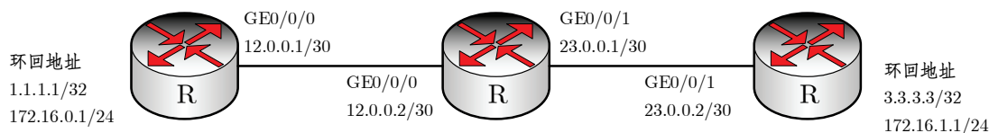
网络拓扑图
