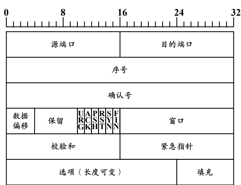
题 47-b 图 TCP 段头结构
