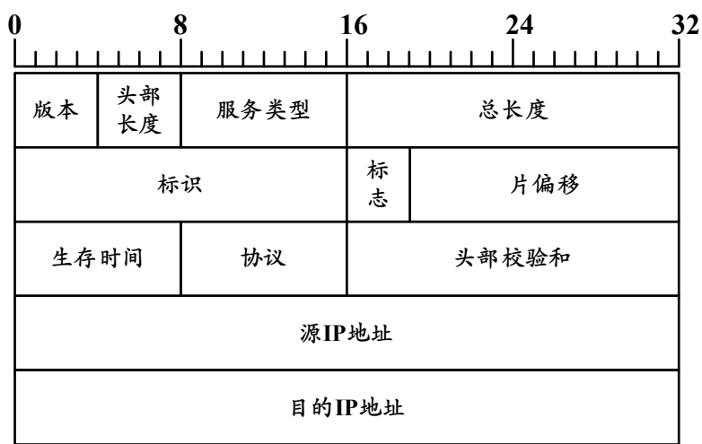
题 47-a 图 IP 分组头结构
