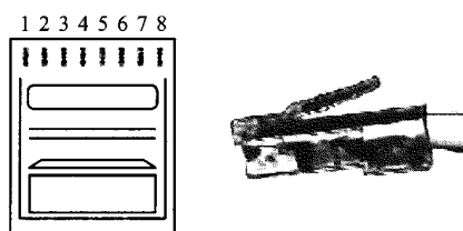
图 2.6 水晶头
