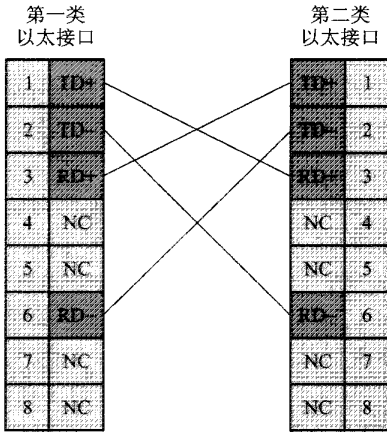
图 2.8 交叉线连接示意图
