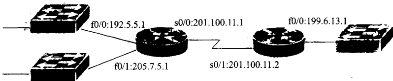
图 5.34 实验用网络拓扑图
