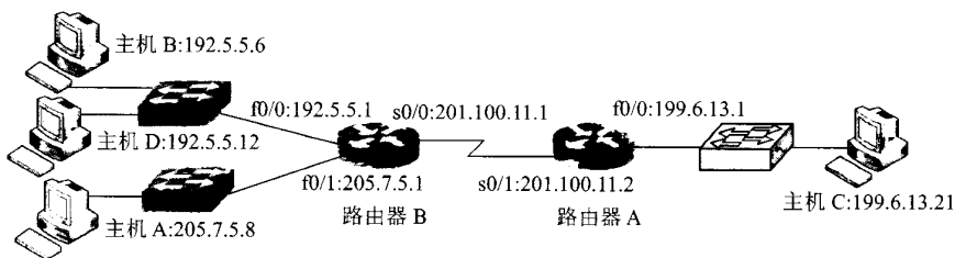
图 5.55 实验拓扑图
