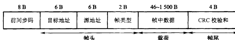
图 3.19 以太网数据帧的格式
