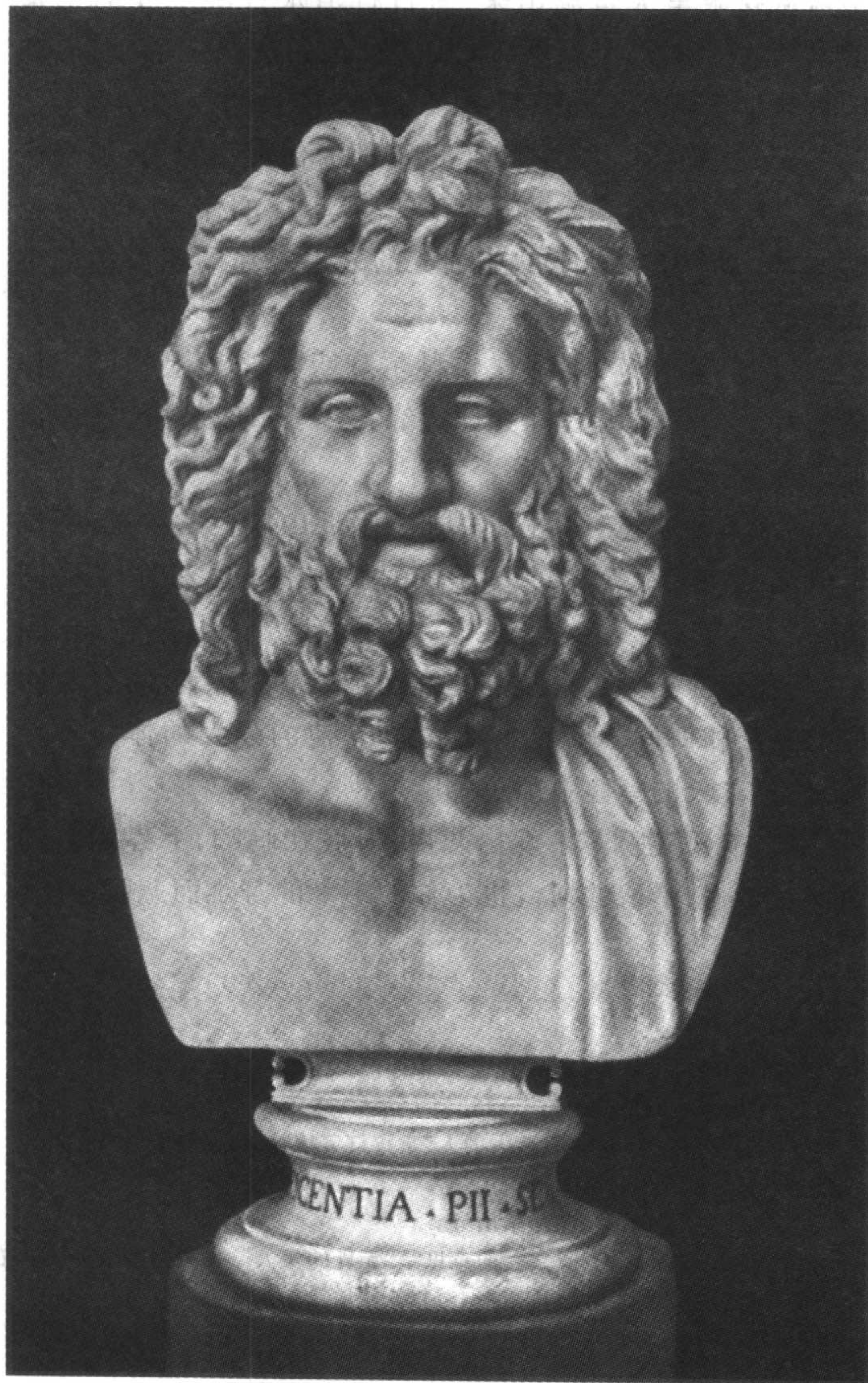
宙斯头像
