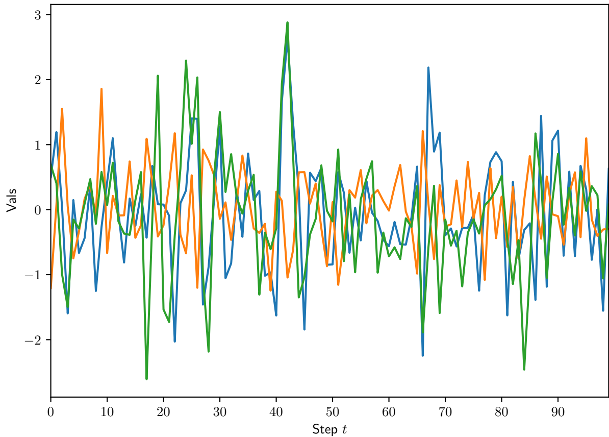
e_t — Latent Noise 4
