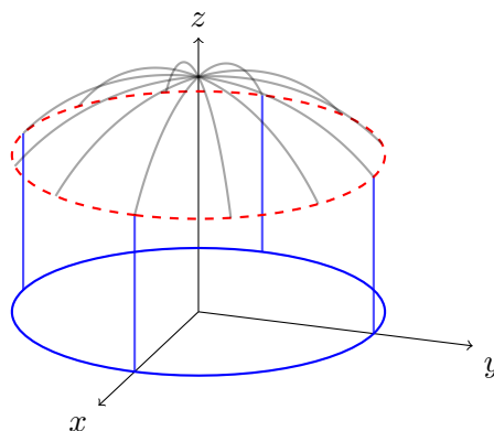
Figur 1.8.: Volum som skal beregnes i Eksempel 1.11
