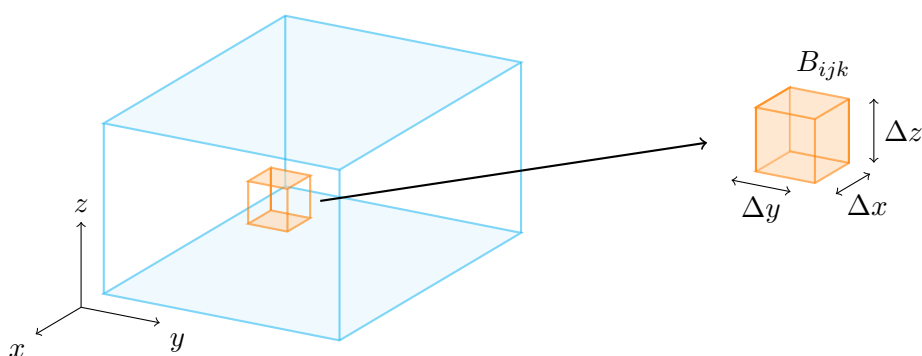
Figur 1.17.: Oppdeling av en boks i små bokser
