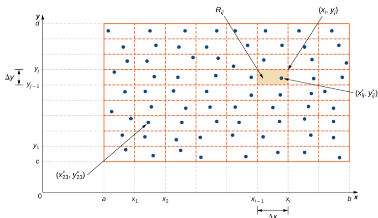
Figur 1.11.: Gitter for integrasjon. Kilde: [SH]:CC BY-NC-SA 4.0.
