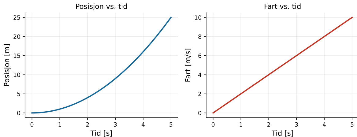
Figur 1.3: Posisjon og fart som funksjon av tid for konstant akselerasjon a = 2.0 \text{ m/s}^2 , v_0 = 0 .
