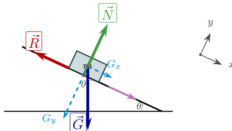
Figur 4.10: Krefter på en kloss som sklir nedover et skråplan. Normalkraften \vec{N} peker normalt ut fra planet, tyngdekraften \vec{G} peker rett ned (med komponenter G_x , G_y langs og normalt på planet), og friksjonskraften \vec{R} peker opp langs planet siden klossen beveger seg ned. Koordinatsystem: x nedover langs planet, y normalt ut.
