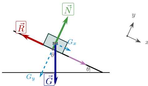
Figur 4.12: Krefter på en kloss på et skråplan. Tyngdekraften \vec{G} dekomponeres i G_x (langs planet) og G_y (normalt på planet). Koordinatsystem: x nedover langs planet, y normalt ut.
