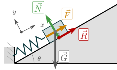
Figur 4.11: Kloss på skråplan ( \theta = 30 ) holdt av fjær \vec{F} og friksjon \vec{R} . Koordinatsystem: x opp langs planet, y normalt ut.
