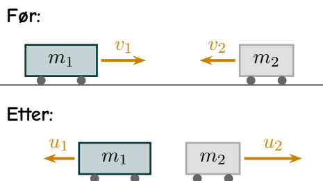
Figur 5.14: To vogner med ulik masse kolliderer elastisk. Positiv retning er mot høyre.
