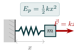
Figur 5.6: Komprimert fjær med kompresjon x . Fjærkraften F = kx skyver klossen vekk. Arbeidet W = \frac{1}{2}kx^2 er lagret som elastisk potensiell energi.
