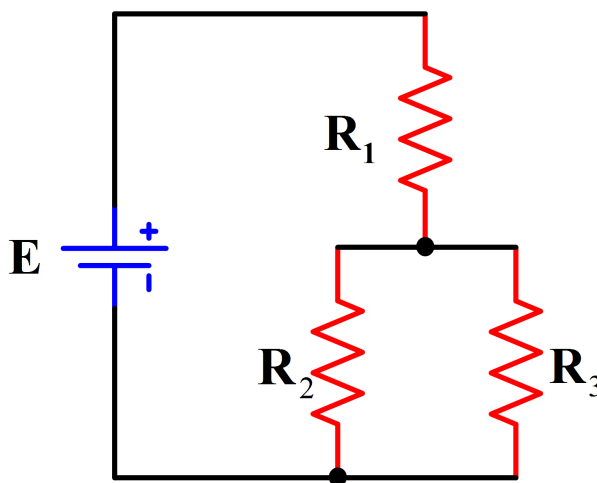
Figur 9.9: Tegning av Krets 1
