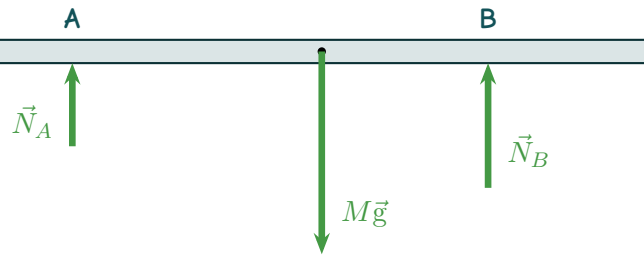
Figur 6.4: Kreftene som virker på bjelken.
