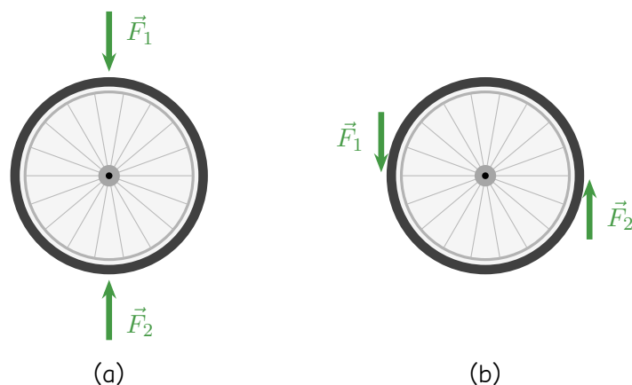
Figur 6.2: Et sykkelhjul som kan rotere fritt om akselen, påvirket av to like store og motsatt rettede krefter, \vec{F}_1 og \vec{F}_2 . (a) Kraftene virker på toppen og bunnen av hjulet og peker rett mot hverandre: hjulet blir stående i ro. (b) De samme kreftene virker i stedet på venstre og høyre side av hjulet: hjulet begynner å rotere, selv om \sum \vec{F} = 0 også her.
