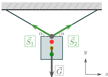
Figur 6.1: Trafikklys i ro. Snorkreftene \vec{S}_1 og \vec{S}_2 danner vinkel \alpha med horisontalen.
