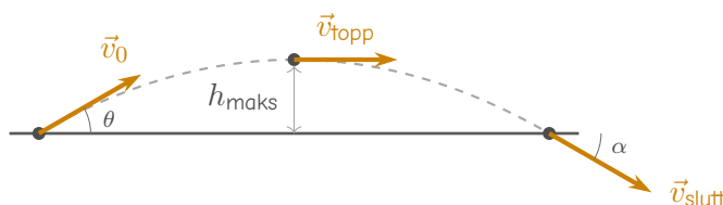
Figur 5.11: Skrått kast uten luftmotstand. I toppunktet peker farten horisontalt.
