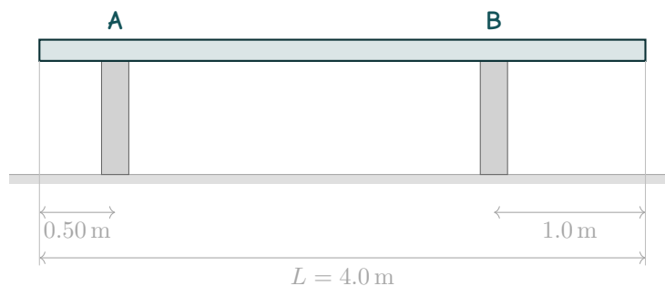
Figur 6.3: En ensartet bjelke som hviler på to søyler, A og B.
