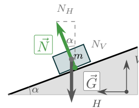
Figur 4.15: Dosert veibane i tverrsnitt. \vec{N} dekomponeres i N_V (opp) og N_H (inn mot sentrum). H -aksen peker inn mot svingensentrummet.
