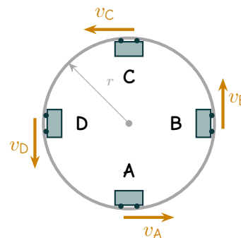
Figur 4.14: Vogn i en vertikal loop på tivoli, sett fra siden. Farten v er tangentiell til sirkelen i alle fire posisjonene.
