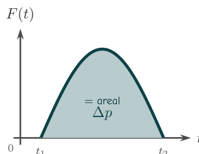
Figur 4.17: Arealet under F(t) -kurven er lik endringen i bevegelsesmengde \Delta p . Kraften varierer typisk under et støt.
