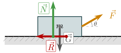
Figur 4.9: Kjelke dradd med kraft \vec{F} i vinkel \theta = 30 over horisontal. Friksjonskraften \vec{R} og normalkraften \vec{N} angriper ved kontaktflaten.
