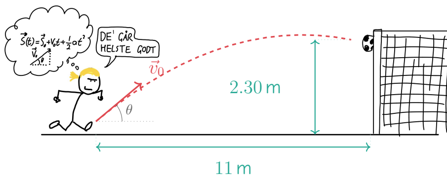
Figur 3.7: Straffespark. Ballens bane er vist med stiptet linje, med utgangsfarten \vec{v}_0 tegnet inn som tangent til banen ved avspark.
