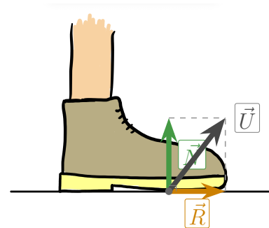
Figur 4.4: En fot som står på bakken. Underlagskraften \vec{U} dekomponeres i normalkraften \vec{N} (vinkelrett) og friksjonskraften \vec{R} (parallelt med underlaget).
