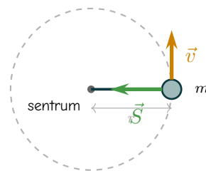
Figur 4.13: Sett ovenfra: ball i sirkelbane. Snorkraften \vec{S} er alltid rettet inn mot sentrum.
