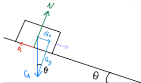
Figur 4.10: Krefter på en kloss som sklir nedover et skråplan. Normalkraften \vec{N} peker normalt ut fra planet, tyngdekraften \vec{G} peker rett ned, og friksjonskraften \vec{R}_k peker opp langs planet siden klossen beveger seg ned.
