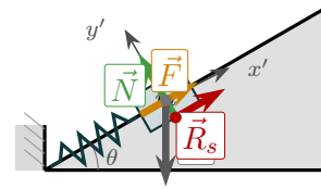
Figur 4.11: Kloss på skråplan ( \theta = 30 ) holdt av fjær \vec{F} og friksjon \vec{R}_s . Koordinatsystem: x' opp langs planet, y' normalt ut.
