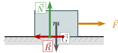
Figur 4.5: Krefter på et objekt som skyves horisontalt. Friksjonskraften \vec{R} virker alltid motsatt av bevegelsesretningen.
