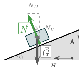
Figur 4.14: Dosert veibane i tverrsnitt. \vec{N} dekomponeres i N_V (opp) og N_H (inn mot sentrum). H -aksen peker inn mot svingssentrummet.
