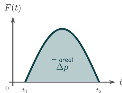
Figur 4.16: Arealet under F(t) -kurven er lik endringen i bevegelsesmengde \Delta p . Kraften varierer typisk under et støt.
