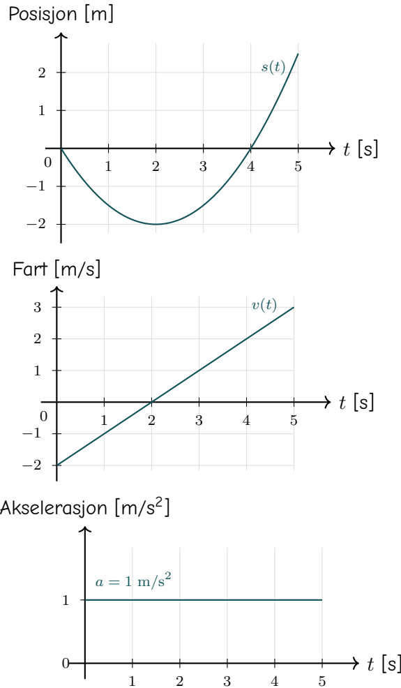
Figur 3.5: Posisjon, fart og akselerasjon ved konstant akselerasjon ( s_0 = 0 , v_0 = -2 m/s, a = 1 m/s²).
