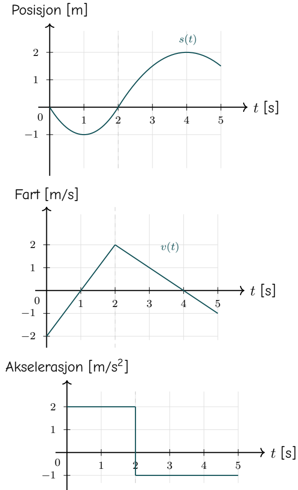
Figur 3.6: Posisjon, fart og akselerasjon ved varierende akselerasjon ( s_0 = 0 , v_0 = -2 m/s; a_1 = 2 m/s² for t \in [0, 2] s og a_2 = -1 m/s² for t \in [2, 5] s).
