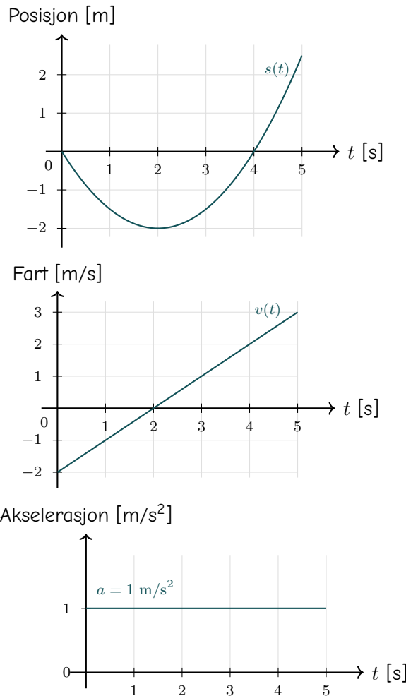
Figur 3.5: Posisjon, fart og akselerasjon ved konstant akselerasjon ( s_0 = 0 , v_0 = -2 m/s, a = 1 m/s 2 ).
