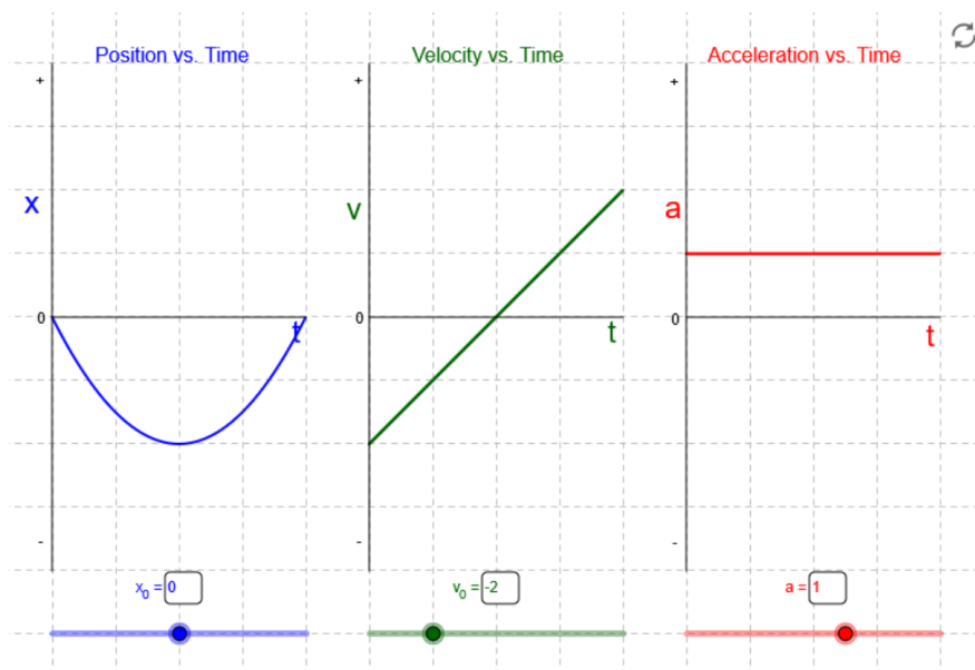
Figur 2.3: Eksempel på posisjon, hastighet og akselerasjonsgraf hvor akselerasjonen er konstant
