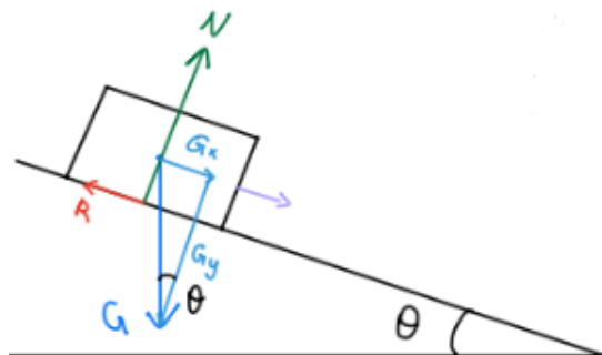
Figur 4.10: Krefter på en kloss som sklir nedover et skråplan. Normalkraften \vec{N} peker normalt ut fra planet, tyngdekraften \vec{G} peker rett ned, og friksjonskraften \vec{R}_k peker opp langs planet siden klossen beveger seg ned.
