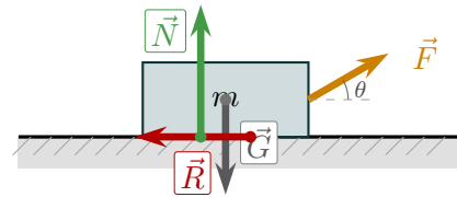
Figur 4.9: Kjelke dradd med kraft \vec{F} i vinkel \theta = 30^\circ over horisontal. Friksjonskraften \vec{R} og normalkraften \vec{N} angriper ved kontaktflaten.
