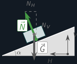
Figure: Dosert veibane i tverrsnitt. \vec{N} dekomponeres i N_V (opp) og N_H (inn mot sentrum).
