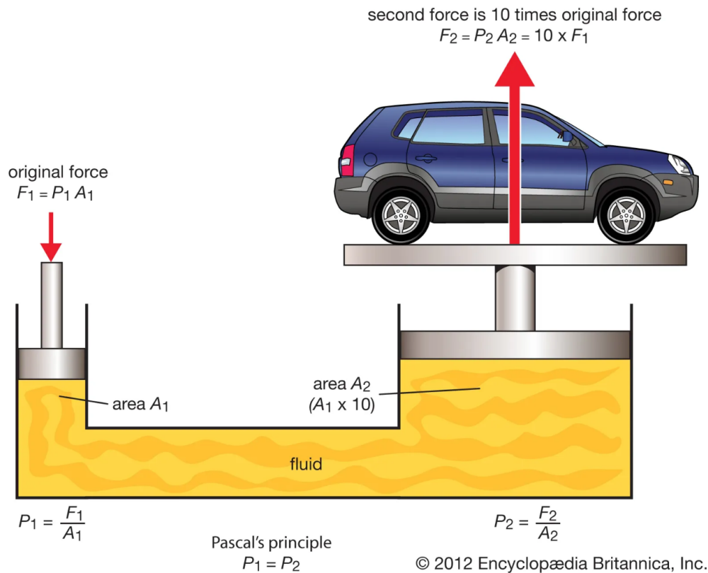
Figur 6.5: Pascals lov i et hydraulisk system. En liten kraft F_1 påføres et lite stempel med areal A_1 , og skaper et trykk som forplanter seg gjennom væsken. Dette trykket løfter en bil ved å bruke et større stempel med areal A_2 , som resulterer i en større kraft F_2 .
