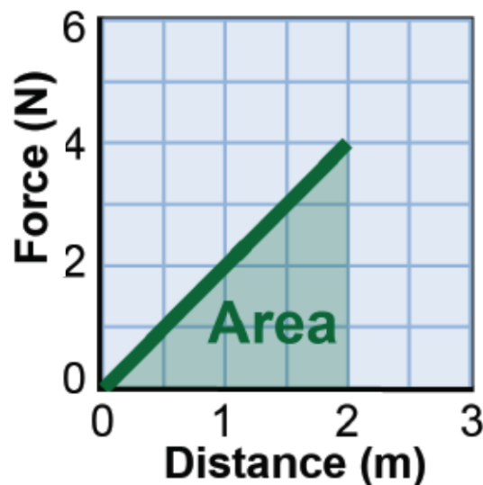
Figur 5.3: Arealet er eksempel på arbeidet for å presse sammen en fjær, når F = k \cdot x og W = \frac{1}{2}kx^2 .
