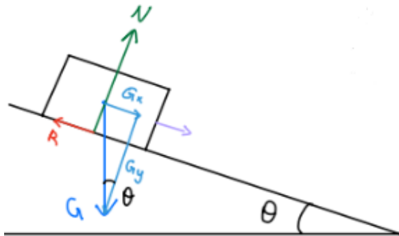
Figur 4.1: Krefter i skråplan
