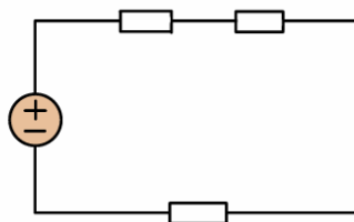
Figur 7.7: Motstander i seriekobling
