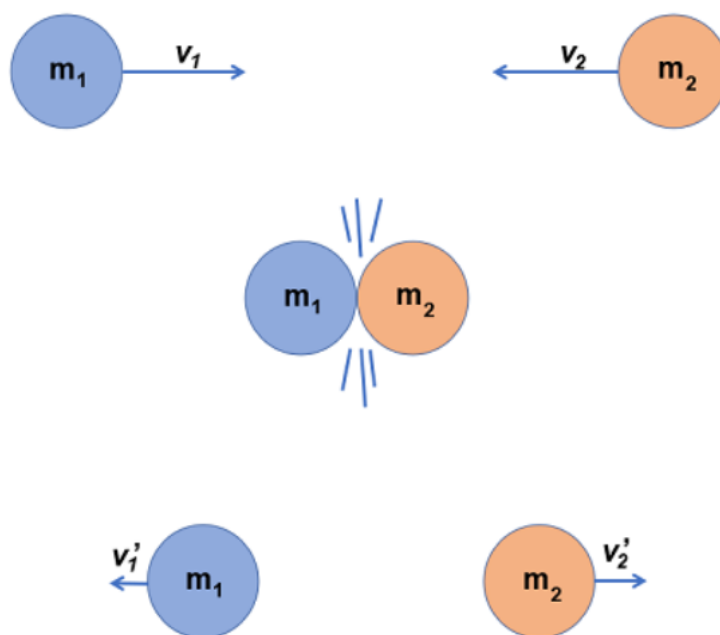
Figur 5.10: Elastisk støt
