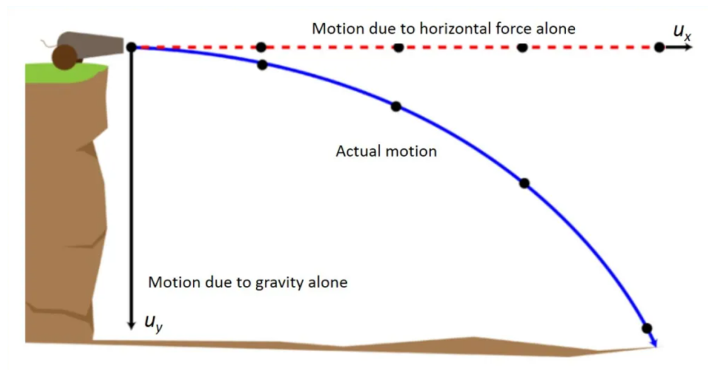
Figur 3.5: Prosjektilbevegelse
