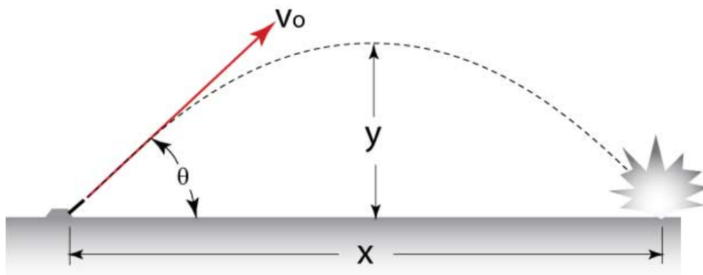
Figur 3.7: Prosjektilbevegelse
