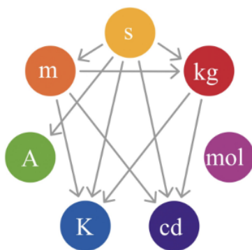
Figur 1.1: SI-enhetene
