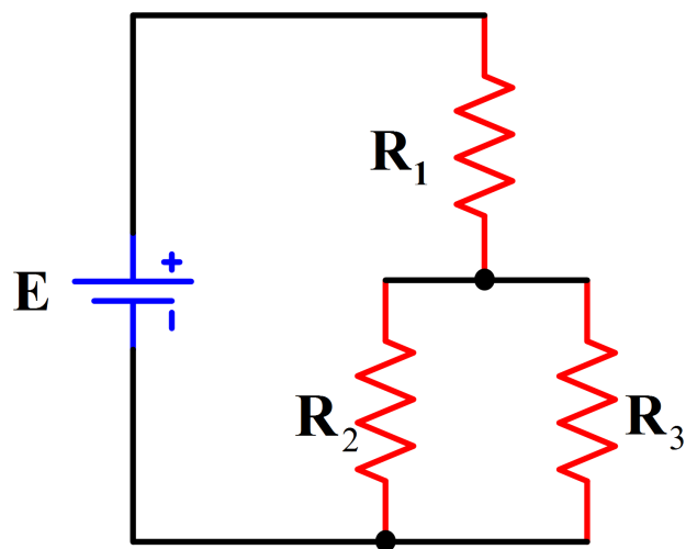
Figur 7.9: Tegning av Krets 1
