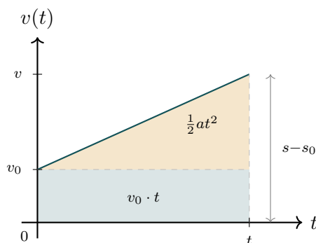
(b) v(t) -grafen. Trapezarealet (rektangel + trekant) er forflytningen: \Delta s = s - s_0 .
