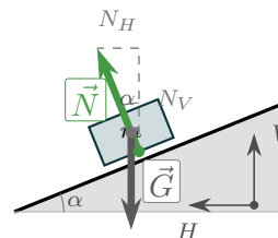
Figur 4.11: Dosert veibane i tverrsnitt. \vec{N} dekomponeres i N_V (opp) og N_H (inn mot sentrum). H -aksen peker inn mot svingssentrummet.
