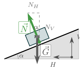
Figur 4.11: Dosert veibane i tverrsnitt. \vec{N} dekomponeres i N_V (opp) og N_H (inn mot sentrum). H -aksen peker inn mot svingssentrummet.
