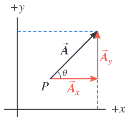
Figur 2.6: Illustrasjon av vektoren \vec{A} og vinkelen \theta .
