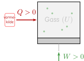
Figur 8.2: Gass i sylinder. Varme Q tilføres fra en varmekilde, og stempelet gjør arbeid W på gassen.
