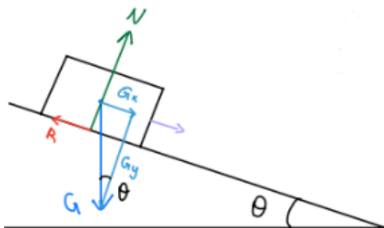
Figur 4.7: Krefter på en kloss som sklir nedover et skråplan. Normalkraften \vec{N} peker normalt ut fra planet, tyngdekraften \vec{G} peker rett ned, og friksjonskraften \vec{R}_k peker opp langs planet siden klossen beveger seg ned.
