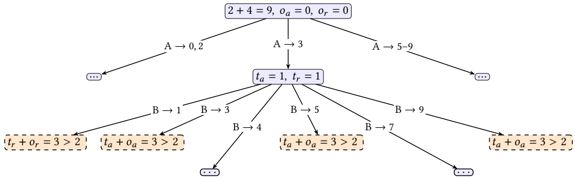
Εικόνα 3: Τμήμα του κατά βάθος δένδρου για τον γρίφο 2 + 4 = 9 και την επιλογή A \rightarrow 3 .
