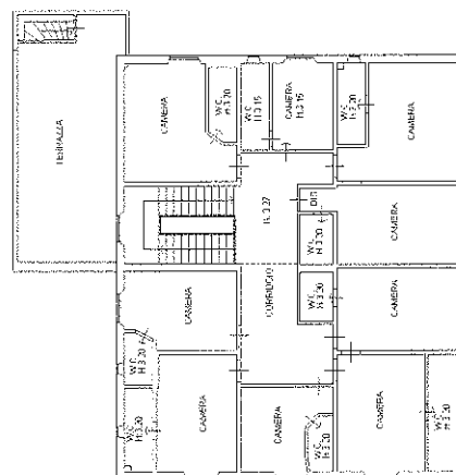
PIANO SECONDO H: 3.37 ML
