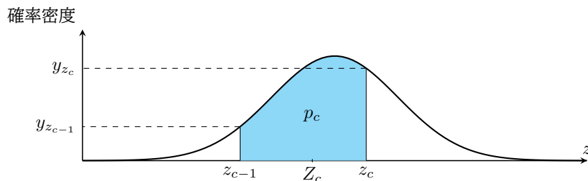
図 A.1 標準正規分布と対応する記号の確認
