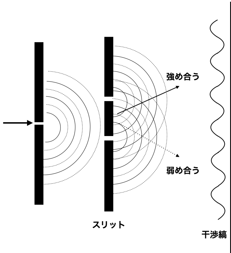
図 2.2 光の干渉縞
