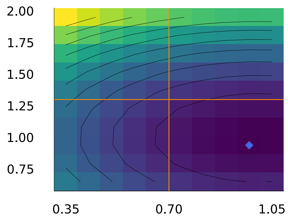
(Param3, Param5)
