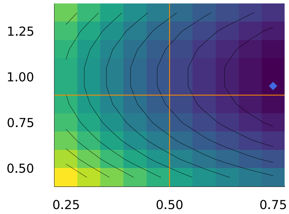
(Param1, Param6)
