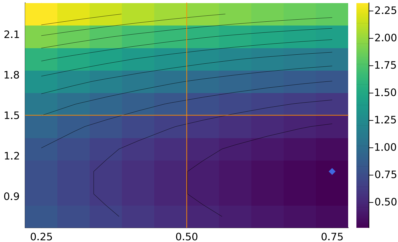
(Param1, Param6)
