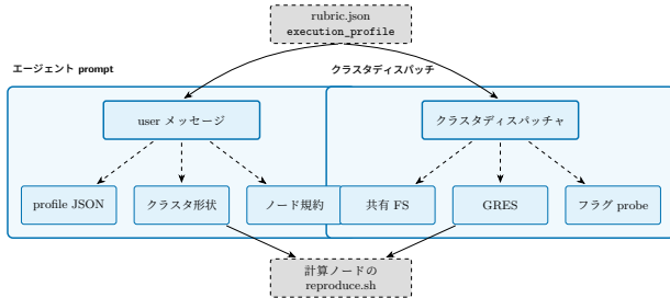
Figure 12: 実行プロファイル契約は単一のルブリック成果物から二つの消費者へ流れる: 複製エージェントのプロンプト (左) とクラスタディスパッチャ (右)。ランタイム probe がディスパッチする資源要求をローカルスケジューラに適応させるため、一つのルブリックが異種クラスタ上で無改変のまま忠実に動く。
