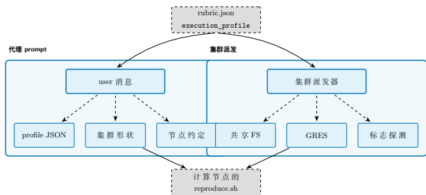
图 12: 执行配置契约从单一评分细则产物流入两个消费方: 复现智能体的提示词 (左) 与集群调度器 (右)。运行时 probe 使派发的资源请求适配本地调度器, 因此一份评分细则在异构集群上无需修改即可忠实运行。
