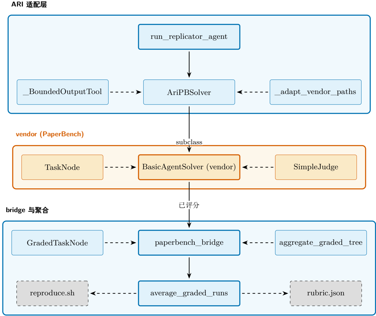
图 5: paper-re 技能的组件。顶行为 ARI 的适配层 (驱动器 + 求解器子类 + 有界工具包装 + 路径适配器); 中行为 vendor 化的 PaperBench 包 (BasicAgentSolver、TaskNode、SimpleJudge); 底行为 bridge, 把按 submission 的 GradedTaskNode 树折叠成单一 rubric.json 得分, 加上 ARI 侧的 reproduce.sh。详见 section 4.4。
