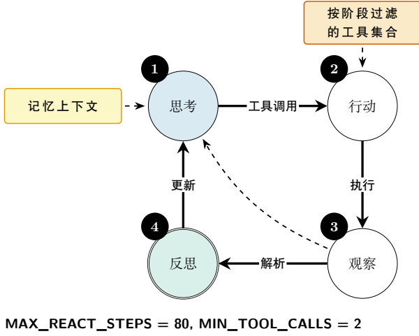
图 9: ReAct 循环。实线为主循环; 虚线反向边表示当观测已闭合开放问题时的提前退出。
