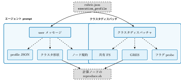
Figure 16: 実行プロファイル契約は単一のルブリック成果物から二つの消費者へ流れる: 複製エージェントのプロンプト (左) とクラスタディスパッチ (右)。ランタイム probe がディスパッチする資源要求をローカルスケジューラに適応させるため、一つのルブリックが異種クラスタ上で無改変のまま忠実に動く。
