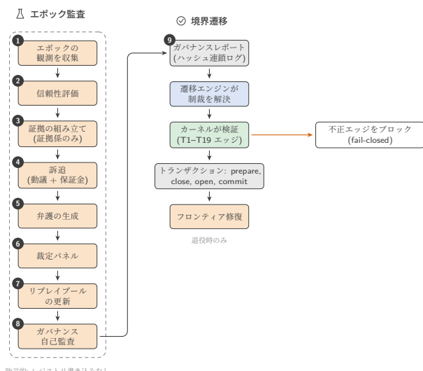
Figure 19: エポック境界パイプライン。九段の監査は助言的であり、レジストリに対しては読み取り専用である; そのレポートはレジストリ遷移エンジンへ供給され、解決された遷移は、四イベントの境界トランザクションがコミットする前に、憲法カーネルによって固定の T1-T19 テーブルに照らしエッジ単位で検証される。不正なエッジは fail-closed でブロックされる——現職のアクティブ集合が引き続き奉仕し、ランは継続する。フロンティア修復が走るのは、コミットされた遷移がコンポーネントまたはプロンプトを退役させた場合に限られる。
