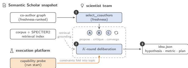
Figure 21: ARI が駆動する VirSci 流の着想生成。 select_coauthors が、凍結された Semantic Scholar スナップショット (SPECTER2 検索インデックスを備えたコーパスと、鮮度順の共著者グラフ) から不均質な科学者チームを編成する; チームはスナップショットに対する検索で基盤づけられた K ラウンドの熟議を行い、実行開始時の能力プローブが、プラットフォームの計測された制約を熟議トピックへ畳み込むため、収束した idea.json は、プラットフォームが実際に計測できる測定だけを約束する。
