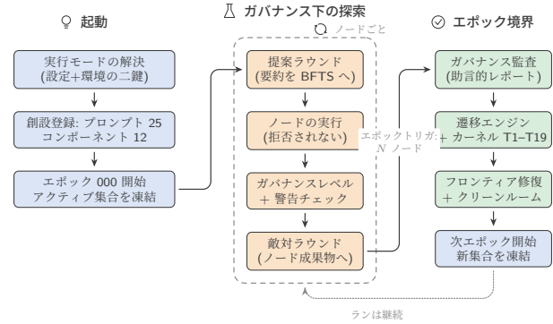
Figure 18: 統治されたランのライフサイクル。起動時に実行モードを解決し、一度限りの創設登録ランザクション (プロンプト 25 件、コンポーネント 12 件) を実行し、創設アクティブ集合をエポック 000 として凍結する。エポックの間、ノード単位のフックが提案を記録し、ガバナンスレベル (固定チェックのみの L0 から完全裁定付きの L3 まで) を割り当て、イベント駆動の敵対ラウンドを実行する; ノードの実行そのものは決して拒否されない。エポックのノード数トリガが発火すると、境界は助言的監査、カーネル検証付きの遷移、そしてクリーンルーム再生成を伴うフロンティア修復を実行し、次エポックのアクティブ集合を凍結して、探索は継続する。
