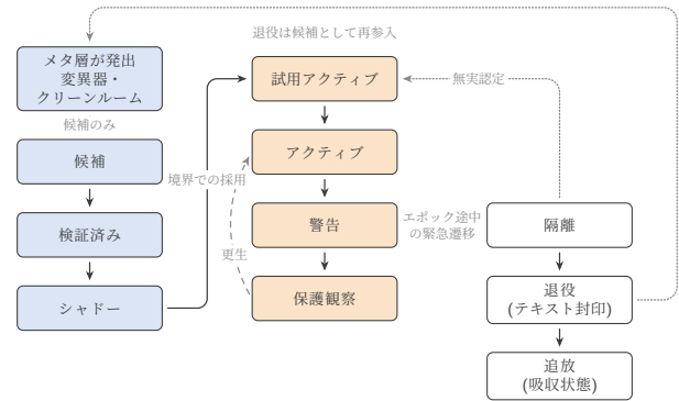
Figure 20: 統治されたプロンプトライフサイクル。メタ層のエージェント (プロンプト変異器; 退役後はクリーンルーム生成器) は候補だけを発出する。候補は六段の検証のはしご (静的、憲法、スキーマドライラン、敵対的ブルに対するリプレイ、アンカー、シャドー) を登り、エポック境界において遷移エンジンによってのみ採用されて、試用として奉仕に入る。制裁は警告、保護観察を経て降下する；強調されたエッジは、唯一のエポック途中遷移である緊急隔離 (T16) である。退役したプロンプトのテキストは封印され、その役割は、クリーンルームによる置き換えが新しい候補としてライフサイクルへ再参入するまで、ベースラインのフォールバックが務める。候補およびシャドーから退役への拒否エッジ (T2、T5) は、明瞭さのため省略した。
