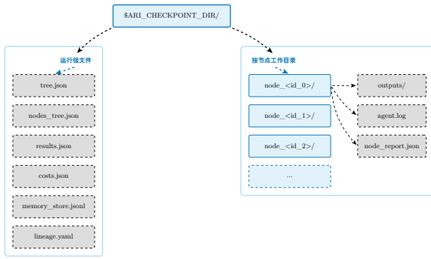
图 6: 检查点目录布局。运行级文件 (左带) 由编排器写入; 按节点工作目录 (右带) 保存一次 BFS 扩展内产生的产物。复现一次运行就是「针对此目录重跑」, 该布局保证不需要其他状态。
