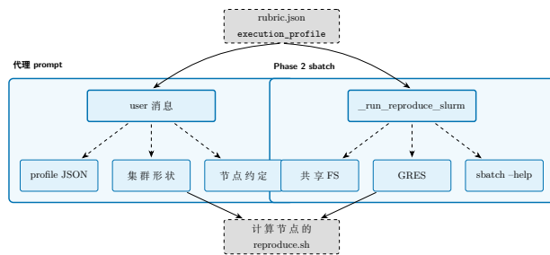
图 10: reproduce_contract.execution_profile 字段从单一 rubric 成果物流入两个消费方: BasicAgent 的 user 消息 (左侧带, 经 _format_hpc_appendix ) 与 Phase 2 sbatch 调度器 (右侧带, 经 _run_reproduce_slurm )。三个运行时探测把发出的标志集适配到本地 SLURM 部署, 因此同一份 rubric 可在异构集群上不加修改地忠实调度。
