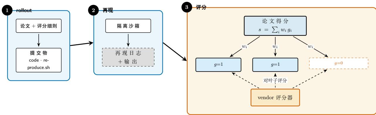
图 14: 将 PaperBench 复现路径表示为三个可组合阶段。智能体的 rollout 把论文及其评分细则转化为 submission(代码与再现脚本);reproduce 在隔离沙箱中执行该 submission, 捕获再现日志及其输出;grade 按加权评分细则树为 submission 评分, 其中 vendor 评分器为每个叶子给出评分 g \in \{0, 1\} , 论文得分是按权重聚合的汇总 s = \sum_i w_i g_i (eq. (8))。
