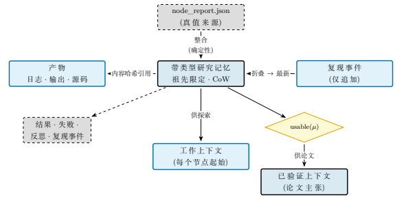
图 10: 可验证研究记忆。对每个节点真值来源 node_report.json 的确定性整合，填充一个按内容哈希索引产物（日志、输出、源码）的带类型存储。复现事件被迫加并折叠为最新状态，准入谓词 \text{usable}(\mu) (eq. (6)) 控制哪些记录进入已验证上下文。同一存储供养两个读者：在下一节点起始注入的工作上下文（探索的继承路径），以及为论文定量主张提供依据的已验证上下文 (section 4.2)。无据的反思可引导探索，但绝不引导论文正文。
