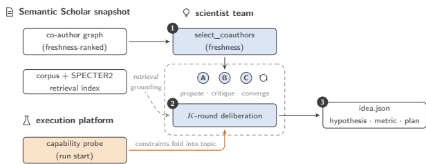
图 17: ARI 所驱动的 VirSci 式想法生成。 select_coauthors 从一份冻结的 Semantic Scholar 快照 (带 SPECTER2 检索索引的语料, 以及按新鲜度排序的合著者图) 组建一支异质的科学家团队; 团队进行以对该快照的检索为奠基的 K 轮研讨, 而一次运行开始时的能力探测把平台被测得的约束折入研讨主题, 使得收敛后的 idea.json 只承诺平台能够进行的测量。
