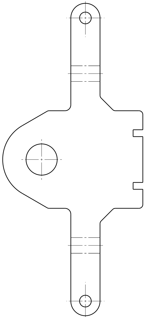
PLANTILLA DE CORTE POR LASER PIEZA: 3.2 ESPESOR: 3.4mm (calibre 10) CANTIDAD: 2 PIEZAS MATERIAL: PLACA ASTM A-36
