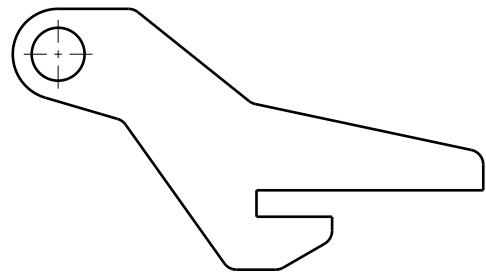
PLANTILLA DE CORTE POR LASER PIEZA: 3.1 ESPESOR: 3.4mm (calibre 10) CANTIDAD: 4 PIEZAS MATERIAL: PLACA ASTM A-36
