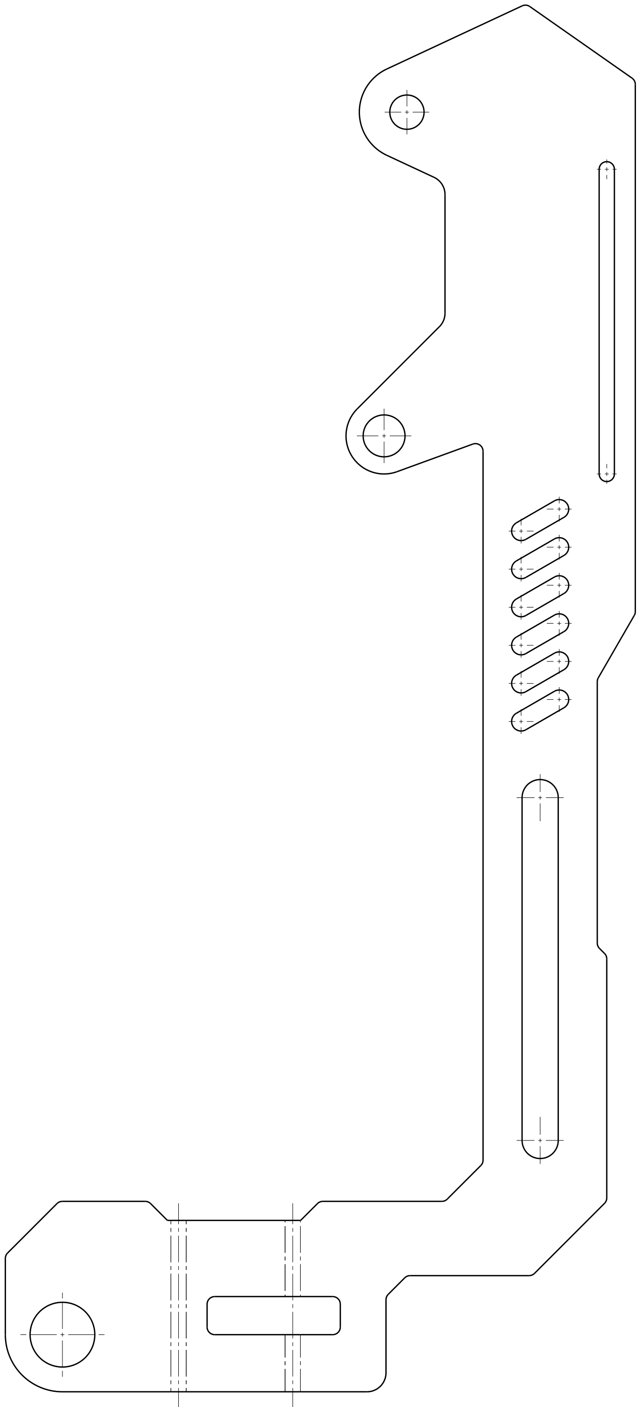
PLANTILLA DE CORTE POR LASER PIEZA: 2 ESPESOR: 3.4mm (calibre 10) CANTIDAD: 2 PIEZAS MATERIAL: PLACA ASTM A-36
