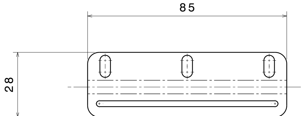
PIEZA DESARROLLADA
