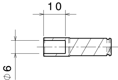
CORTE 0-0
