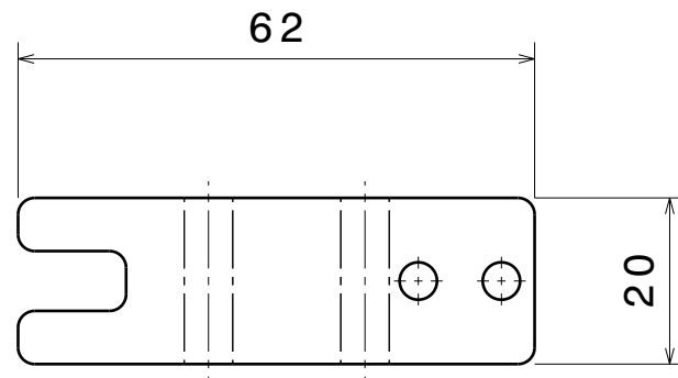
PIEZA DESARROLLADA
