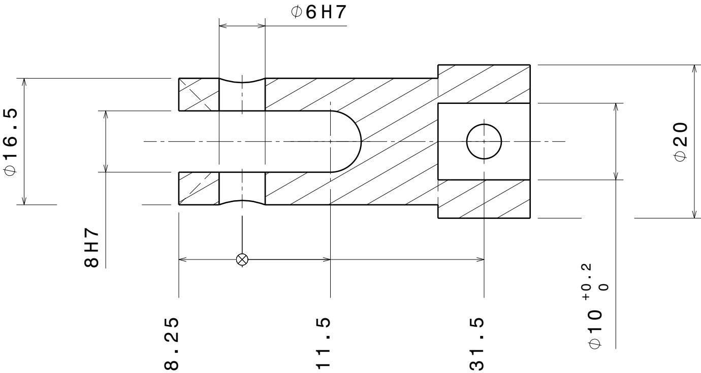
CORTE H-H
