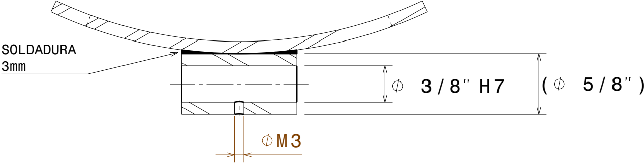
VISTA CORTE SECCIÓN A-A
